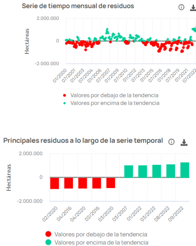
Figura 11. Ejemplo de las diferencias entre el modelo ajustado y los datos observados. Los puntos y barras verdes indican valores de aumento, mientras que los puntos y barras rojas indican valores de disminución en relación a lo esperado por el modelo armónico.
