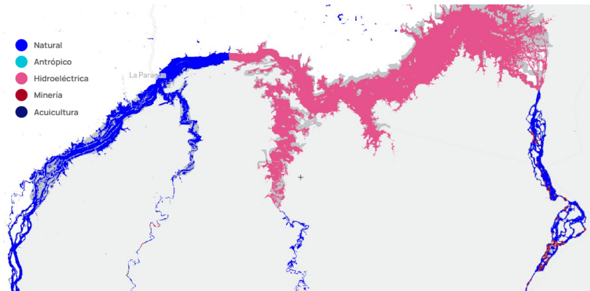
Figura 6. Ejemplos de categorías de cuerpos de agua, estado Bolívar, Venezuela
