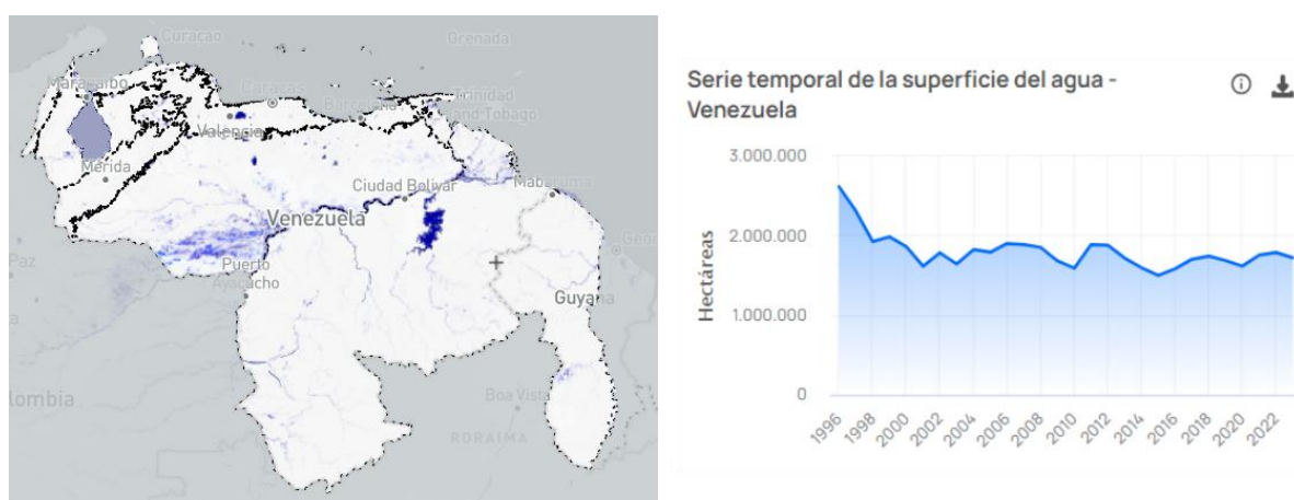
Figura 7. Ejemplo de visualización de los datos de la capa de superficie de agua (mapa y gráfico) en la plataforma de MapBiomas Agua Venezuela.
