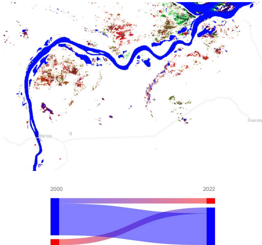
Figura 9. Ejemplo de transición de superficie de agua al sur del río Orinoco, estado Bolívar. El color verde en el mapa indica el incremento de agua en los últimos años debido a la dinámica natural del flujo de agua y cómo este ha cambiado el curso del río; en rojo, se observa dónde ha disminuido el agua debido al mismo fenómeno. El gráfico (azul y rojo) indica las transiciones entre los años seleccionados, de acuerdo al área de superficie mapeada.
