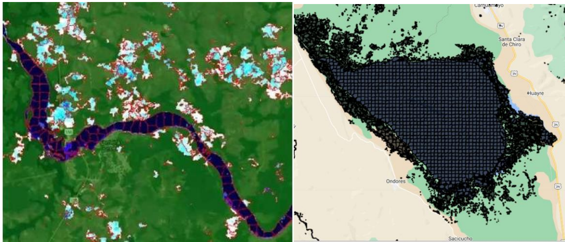
Figura 7. Ejemplos del proceso de segmentación que convierte datos raster (frecuencia mensual dentro de cada año) en una malla de vectores regulares.
