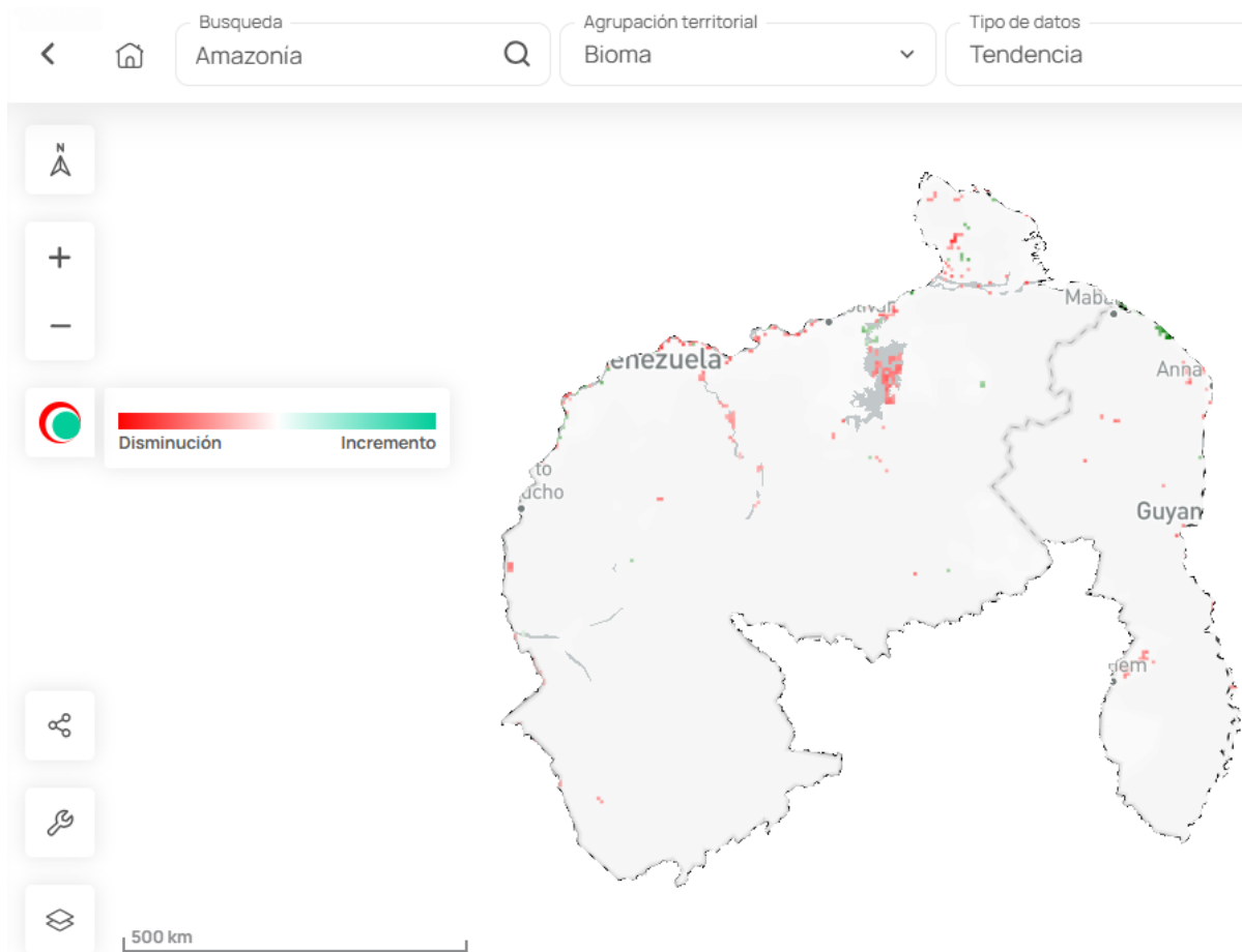
Figura 12. Ejemplo de resultados de cálculo de tendencias en la Amazonia venezolana utilizando la prueba estacional de Mann Kendall. Los datos en rojo indican una disminución, los datos en verde un aumento y los datos en blanco, estabilidad. Sólo se presentan datos con valores significativos.
